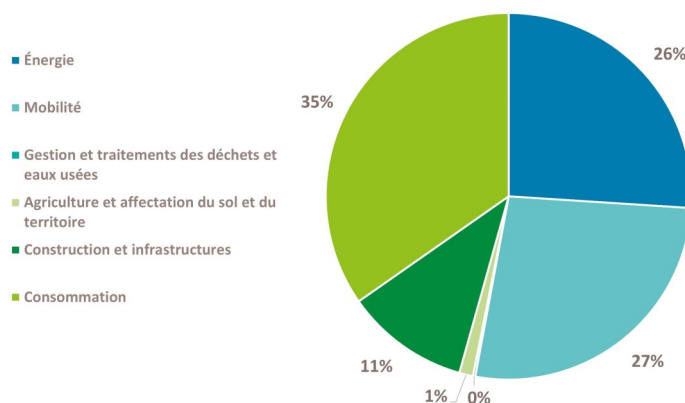
Émissions de gaz à effet de serre pour Etoy, 2019
