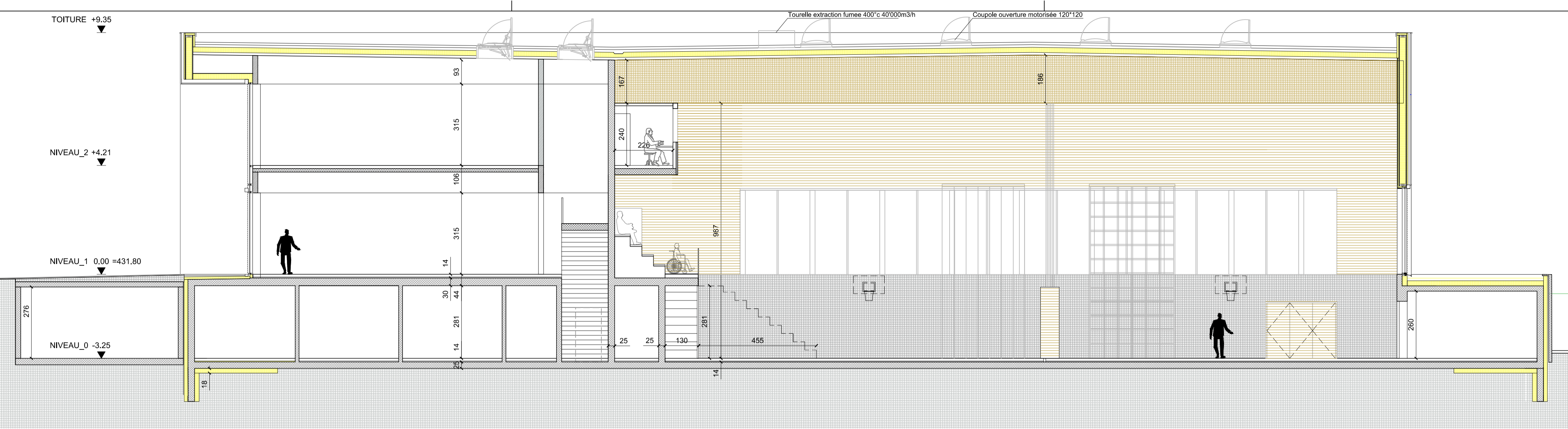
Coupe AA
