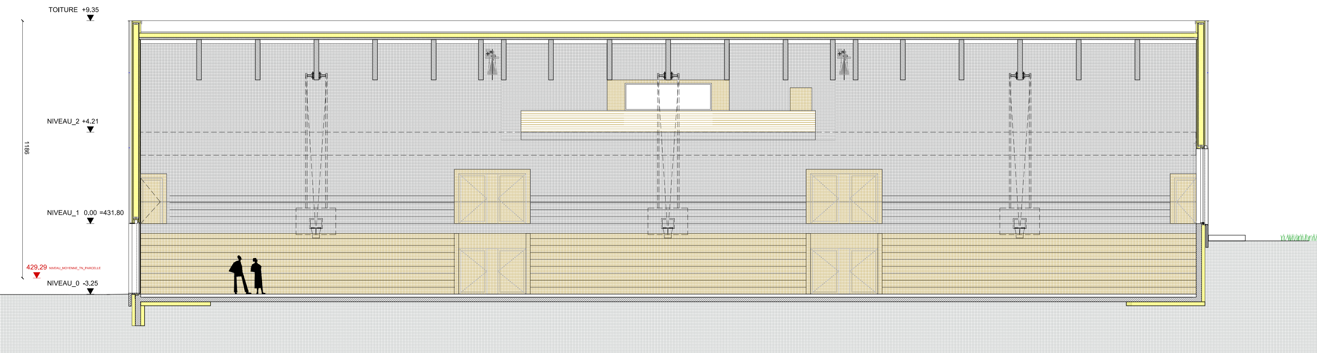
Coupe BB
