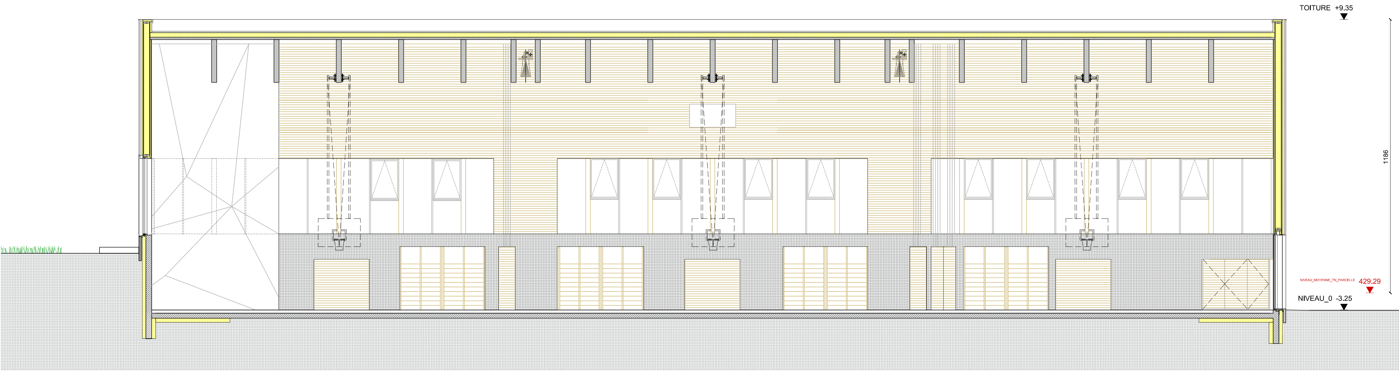
Coupe FF
