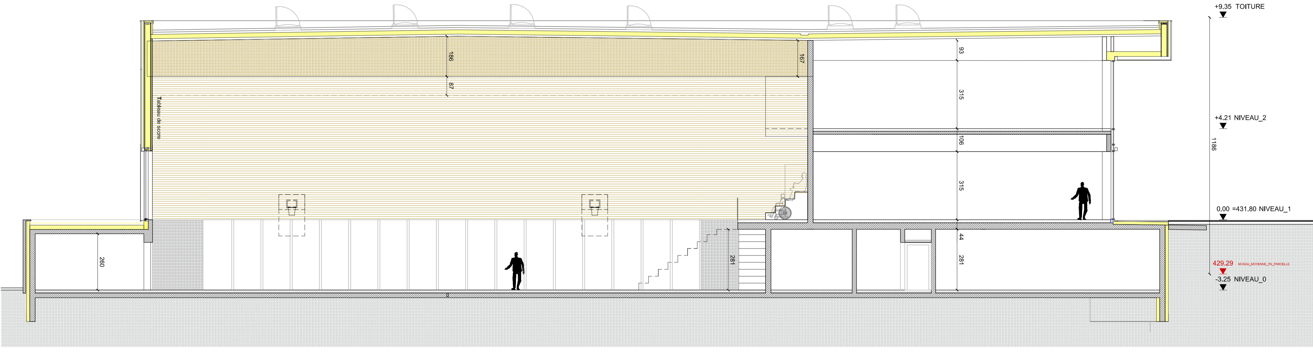
Coupe EE
